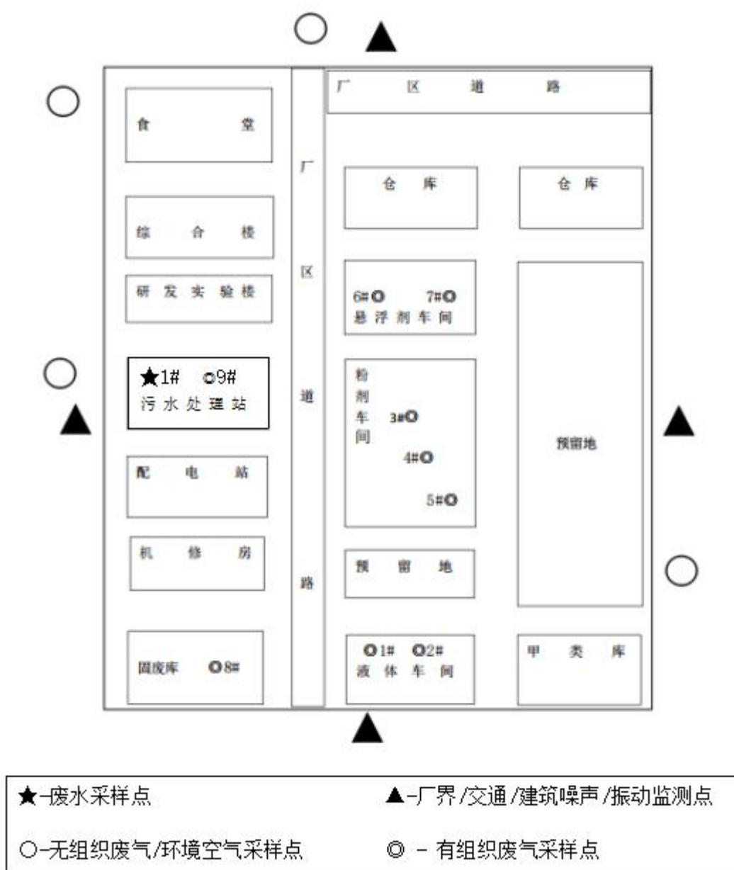
图 1: 废气、粉尘、噪声监测点位示意图
